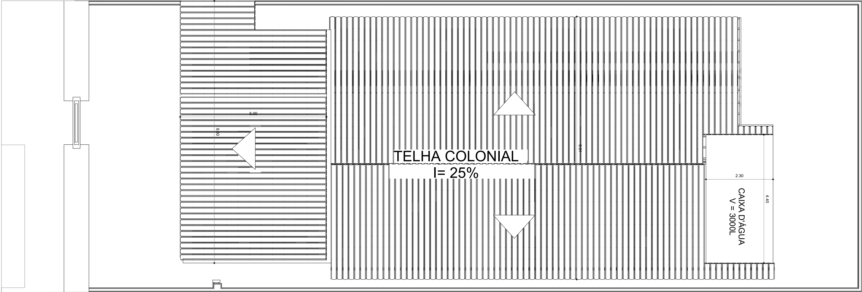
03 PLANTA DE COBERTA ESCALA — 1 : 75
